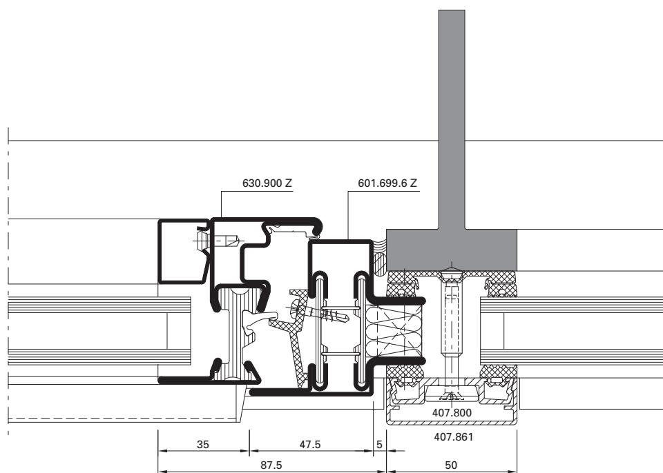
Einsatzelement Fenster Janisol Primo
