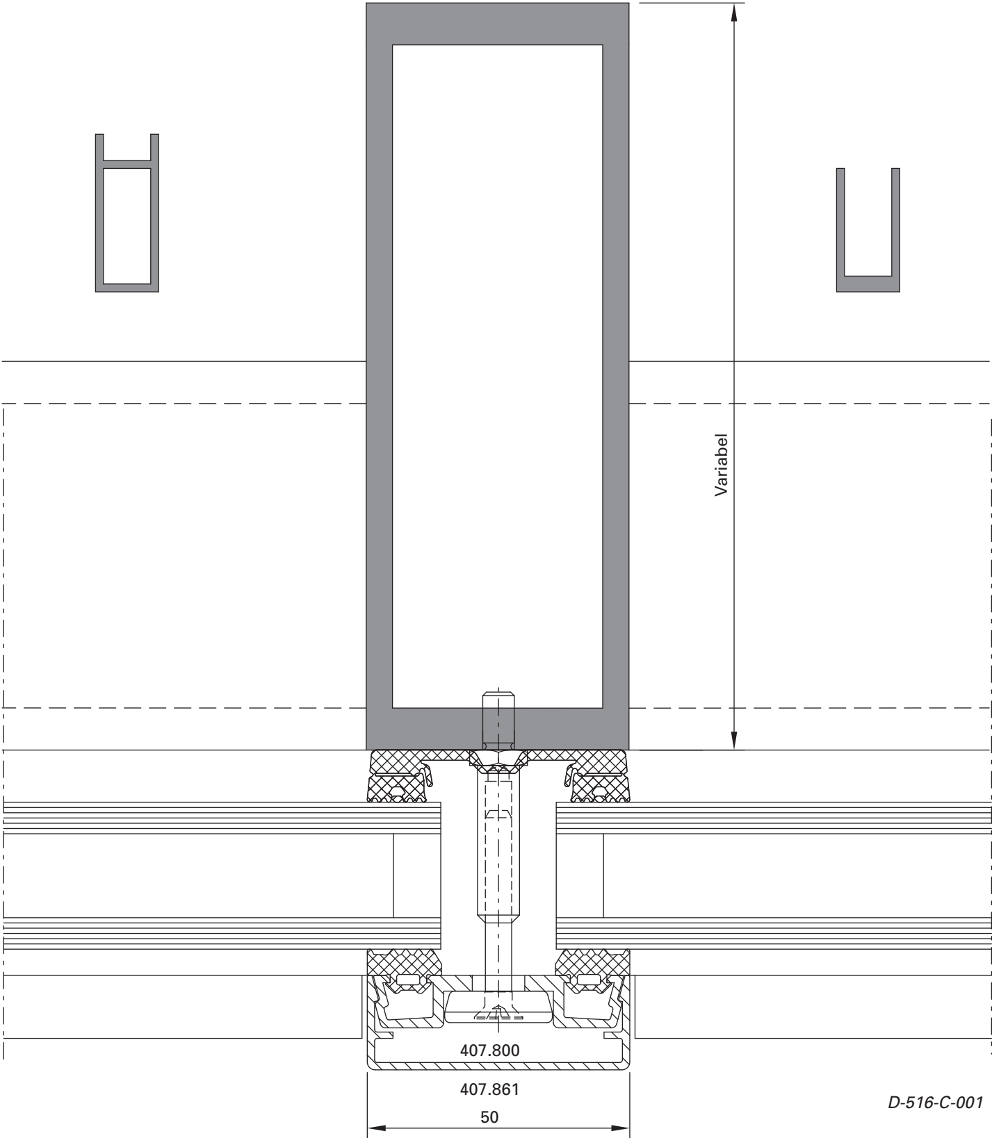
Pfosten-Detail VISS I x tra Ansichtsbreite 50 mm Schraubbolzen
