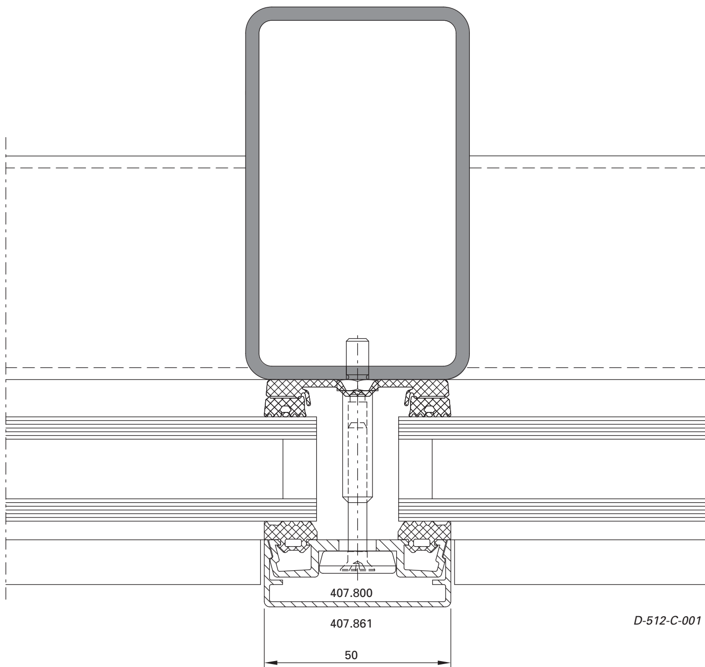
Détail du montant Largeur de face 50 mm Goujon à visser
