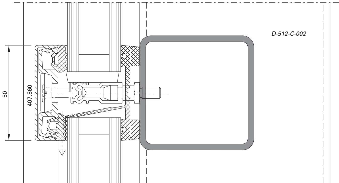
Détail de la traverse Largeur de face 50 mm Goujon à visser
