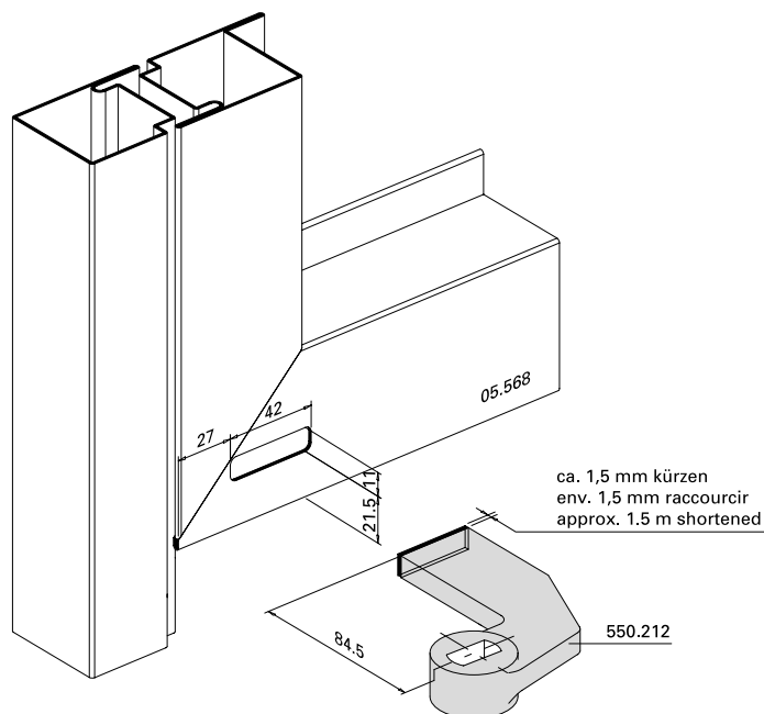
Türhebel 550.212
