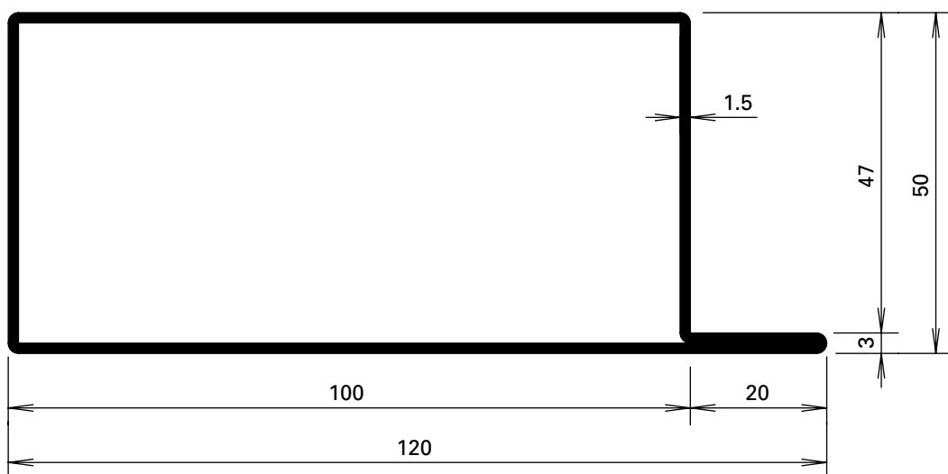
01.596
