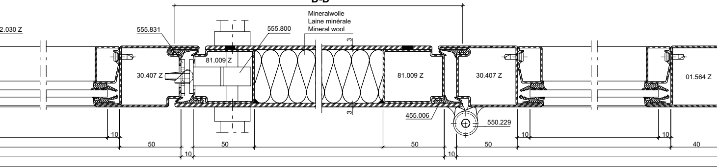
D-D
