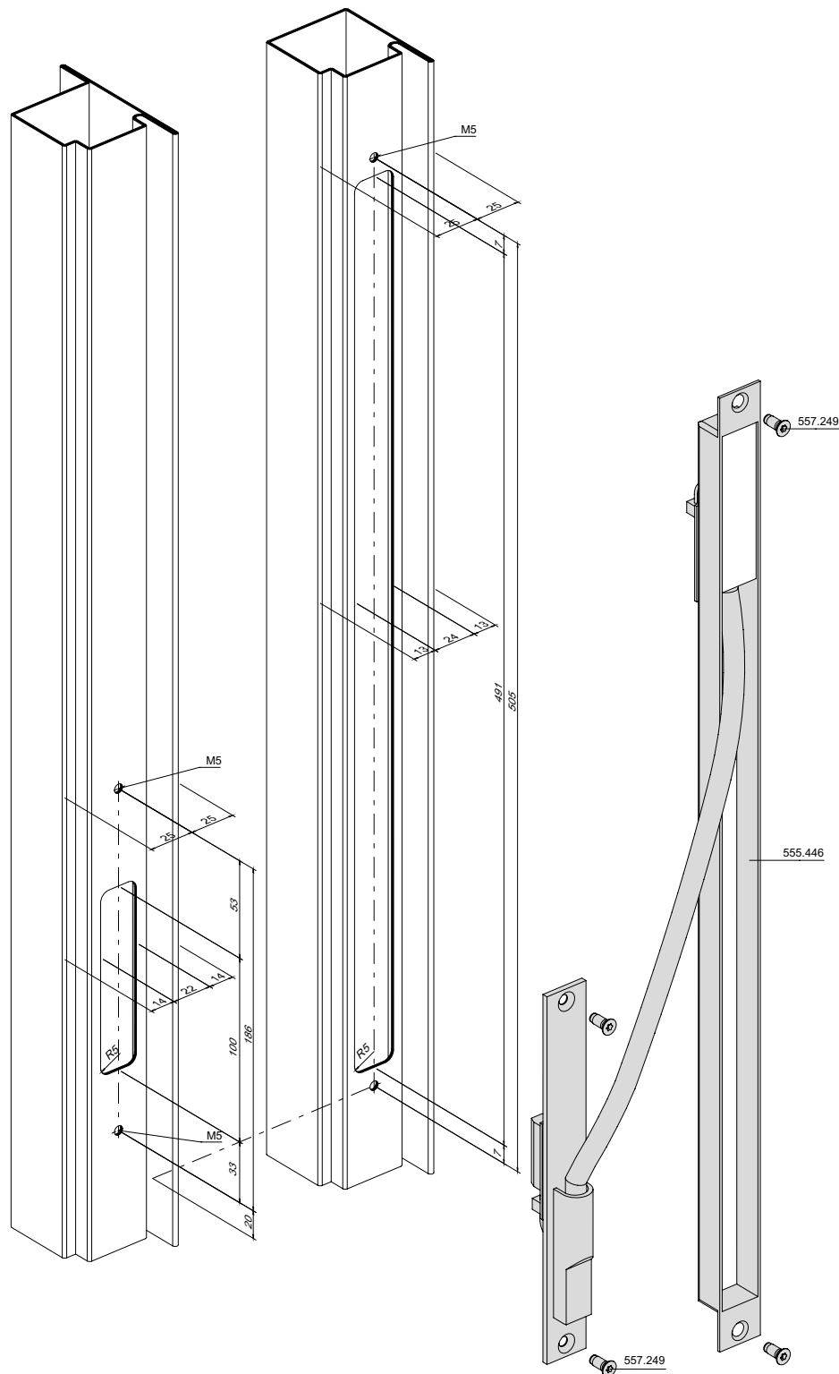
Kabelübergang 555.446 10-polig
