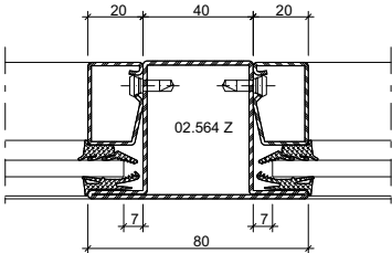
Detail Pfosten/Riegel Détail montant/traverse Detail mullion/transom
