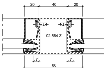
Detail Pfosten/Riegel Détail traverse/montant Detail transom/mullion
