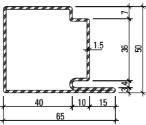
30.007 30.007 Z 30.007.01
