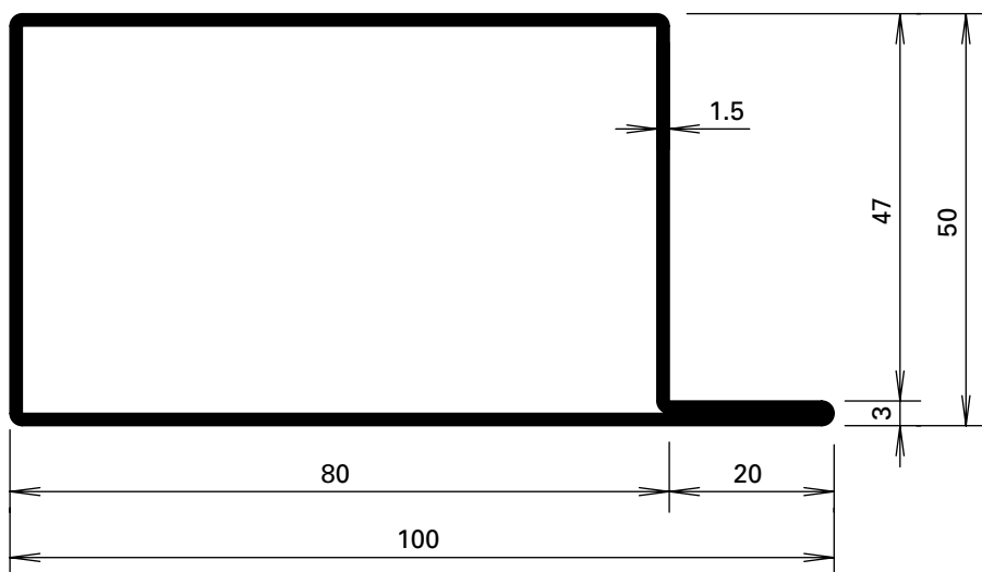
01.592 01.592 Z
