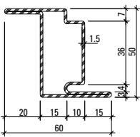
30.406 30.406 Z
