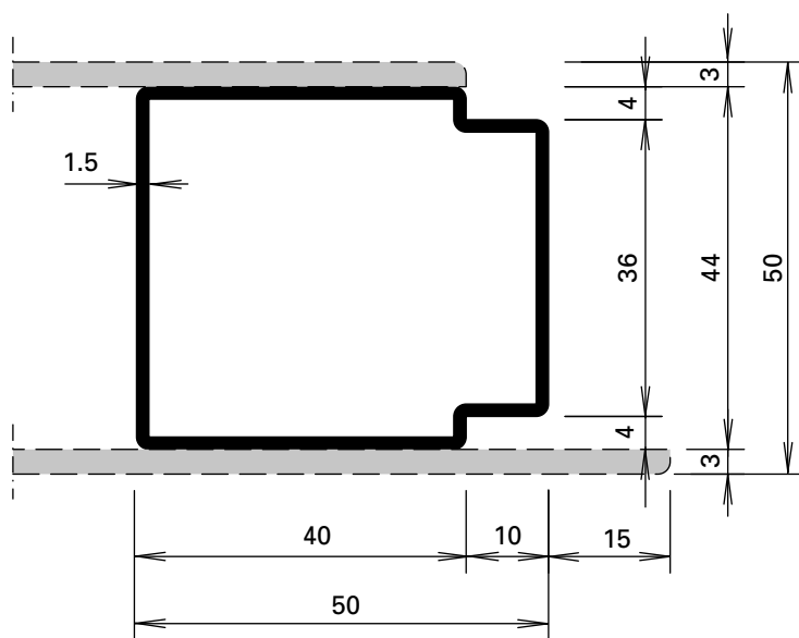
81.009 Z
