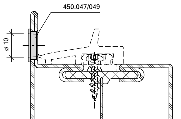
Sitz Entwässerungstülle Ajustement de la douille d'évacuation d'eau Placement of drain pipe
