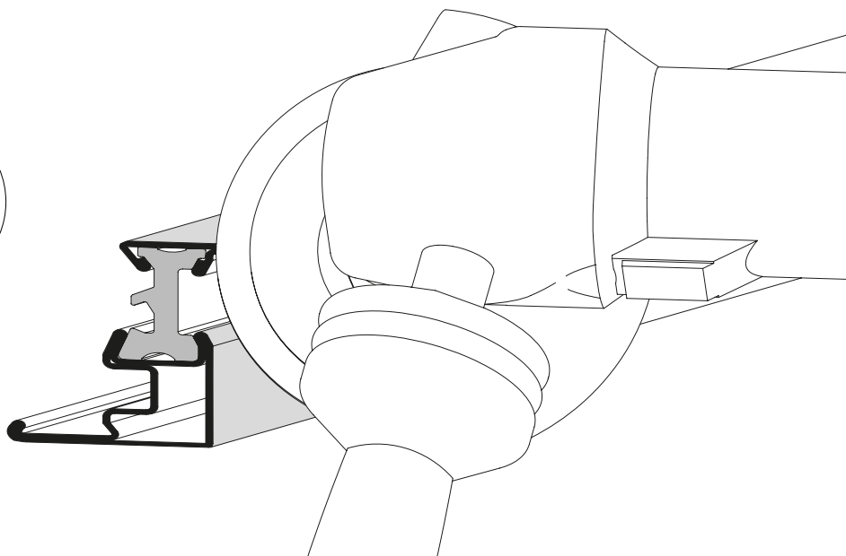
Profile im Schweisssnahtbereich mit Winkelschleifer leicht anschrägen Biseautage léger des profilés dans la zone de la soudure avec une meuleuse d'angle Slightly chamfer the profiles in the area of the weld seam using an angle grinder
