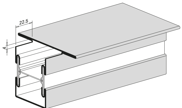
Ausklinkung Riegel auf Stirnseite Entaille traverse en face avant Notching of transom on front
