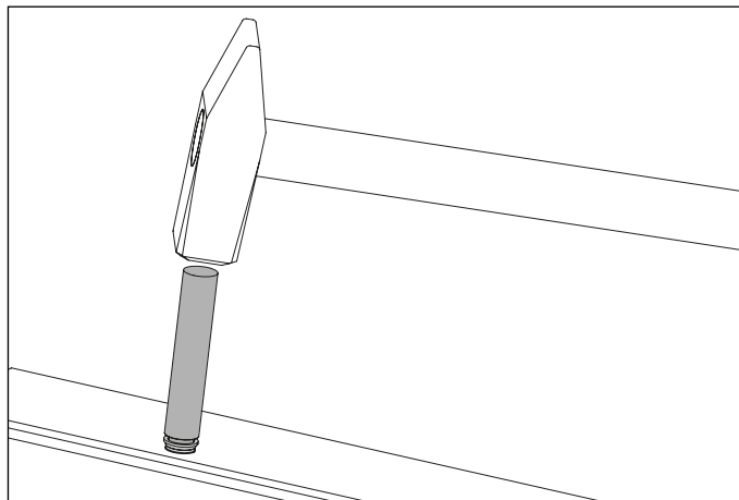
Einschlagen der Tülle mit Montagewerkzeug 499.318 und Stahlhammer (Achtung: Unterlagen verwenden)
