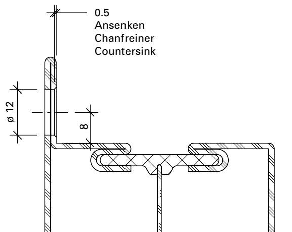
Bohrung und Ansenkung Entwässerungslöcher Perçage et chanfreinage des trous d'évacuation d'eau Drilling and countersinking of drainage holes
