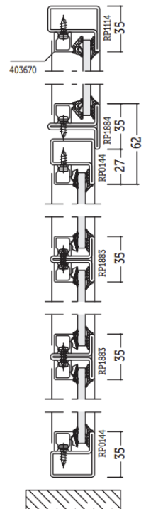
Przekrój/Section C-C
