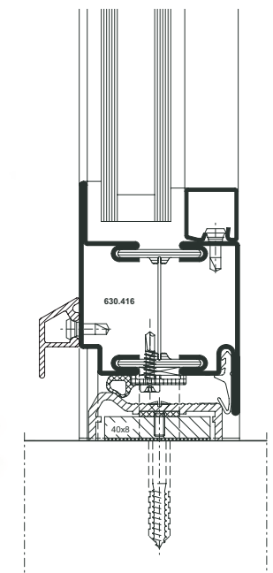
Barrier-free door
