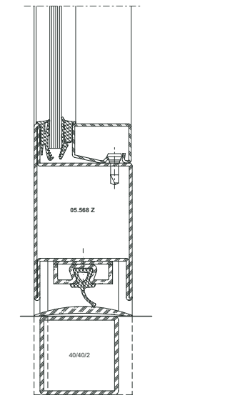
Barrier-free door
