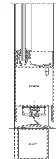
Barrier-free door
