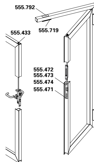
Variante Elektro-Türöffner Variante gâche électrique Version electric strike
